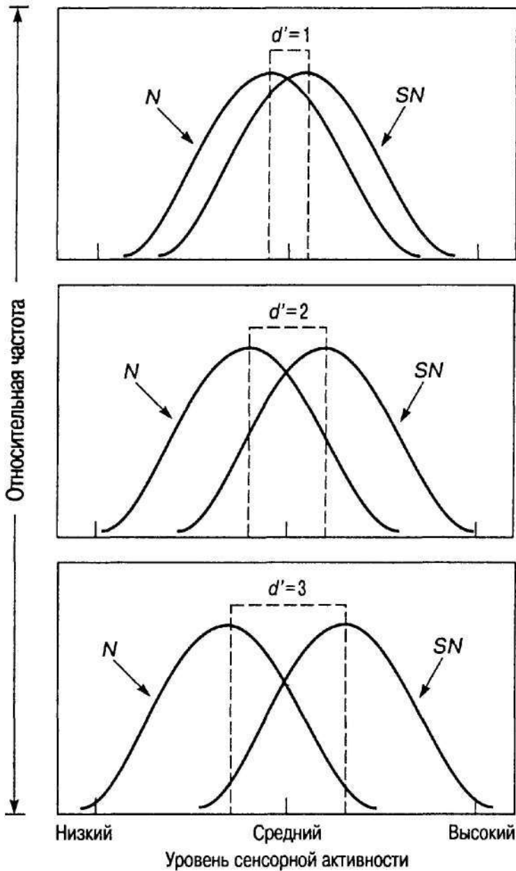
Рис. 2.8. Кривые распределения Ш и СШ для трех РХП, представленных на рис. 2.7. Значение d' изменяется в зависимости от смещения распределения СШ относительно распределения Ш и равно расстоянию между средними значениями Ш и СШ . Для s' = 0 кривые распределения СШ и Ш полностью совпадают. Следовательно, величина d' характеризует интенсивность сигнала и чувствительность к нему наблюдателя, не зависящую от искажения ответа
