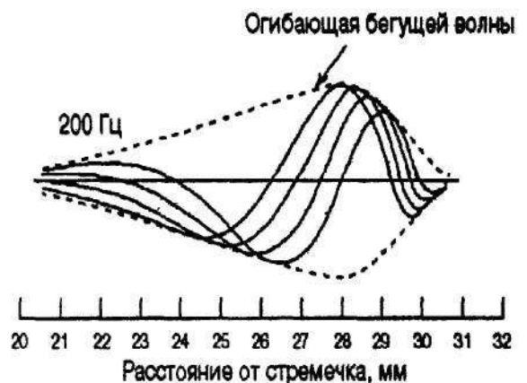
Рис. 12.18. Огибающая тона с частотой 200 Гц
