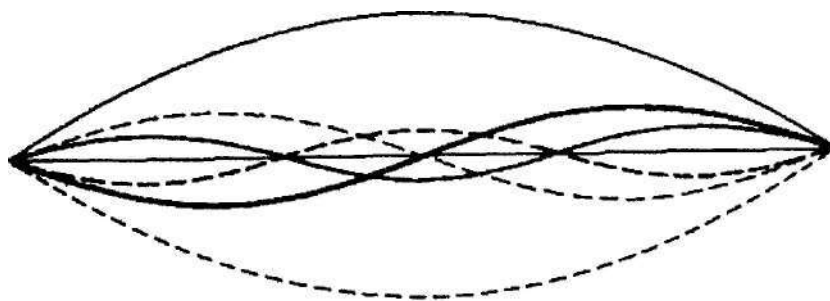
Рис. 12.7. Колебание струны музыкального инструмента
