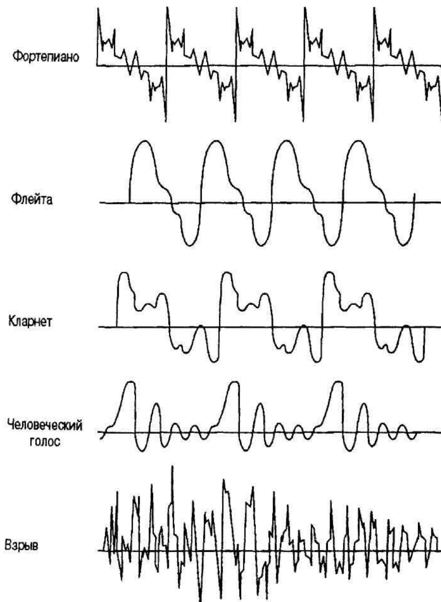
Рис. 12.6. Типичные звуковые волны, соответствующие некоторым звукам
