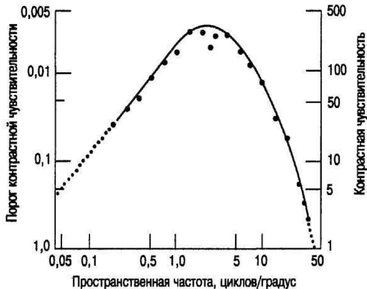
Рис. 6.12. Функция контрастной чувствительности
