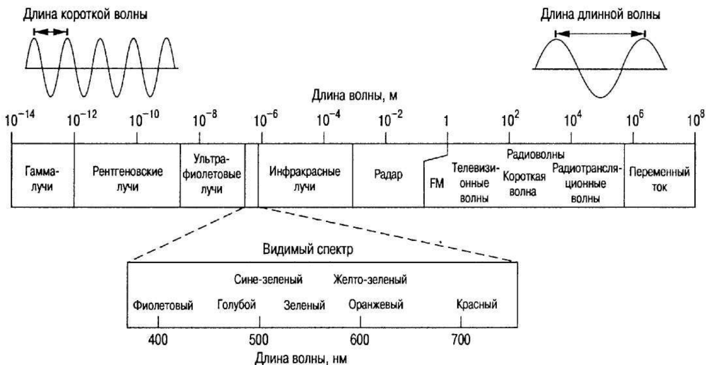
Рис. 3.2. Электромагнитный спектр
