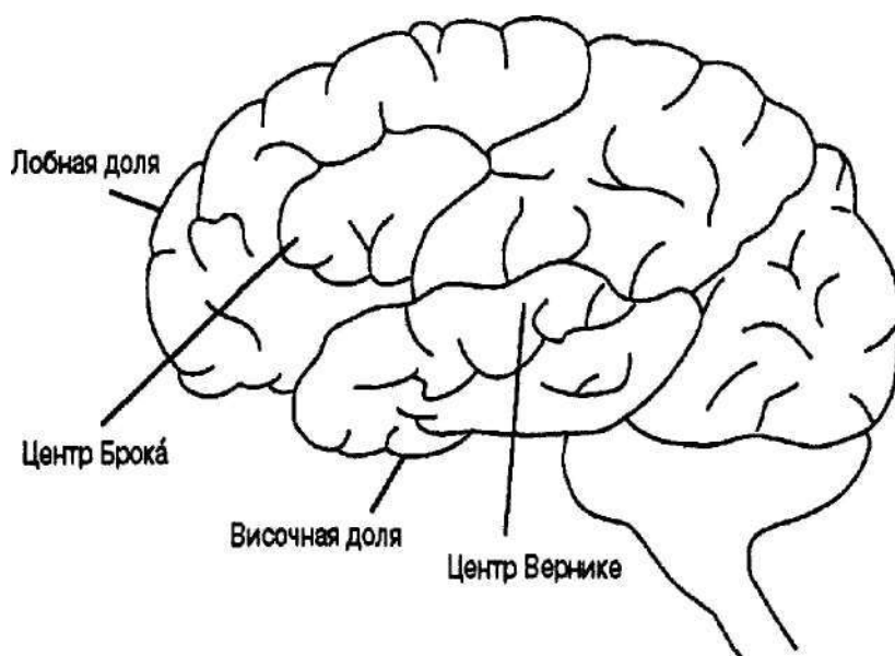
Рис. 14.9. Схематическое изображение левого полушария головного мозга человека
