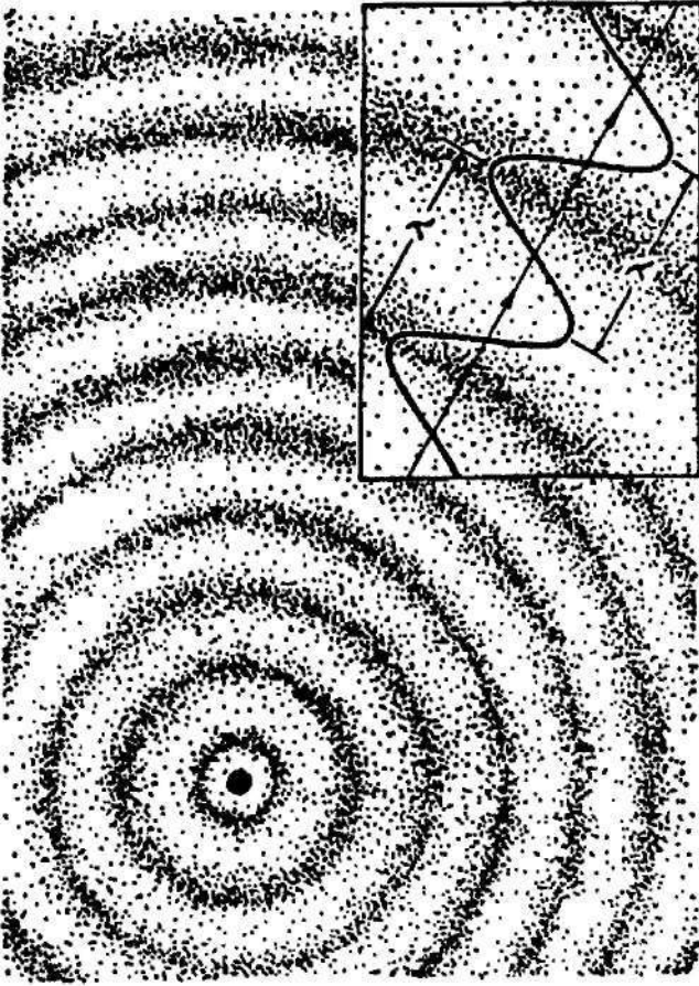
Рис. 12.3. Источник звука представлен в виде центра концентрических окружностей
