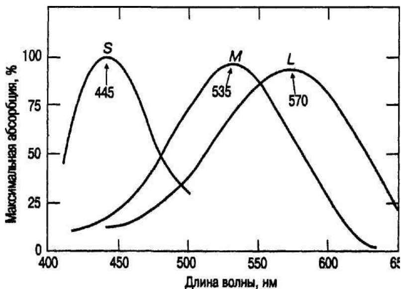
Рис. 5.9. Абсорбционные кривые
