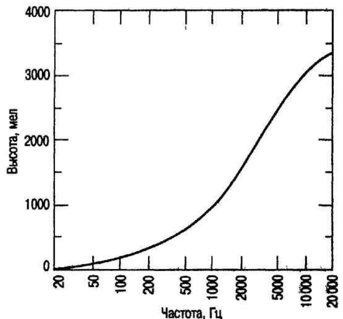
Рис. 13.4. Зависимость высоты тона от его частоты
