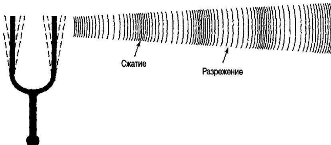
Рис. 12.1. Вибрация камертона
