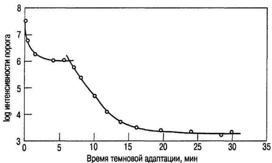
Рис. 4.1. Зависимость величины зрительного порога от времени темновой адаптации. Верхняя часть кривой - колбочковое зрение, нижняя часть - палочковое зрение. (Источник: Hecht & Schlaer, 1938)
