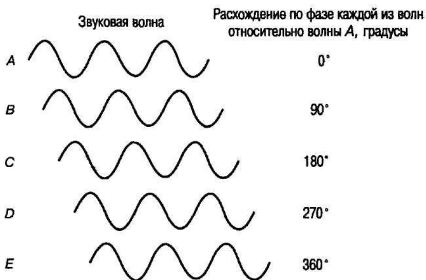
Рис. 12.9. Расхождение звуковых волн по фазе
