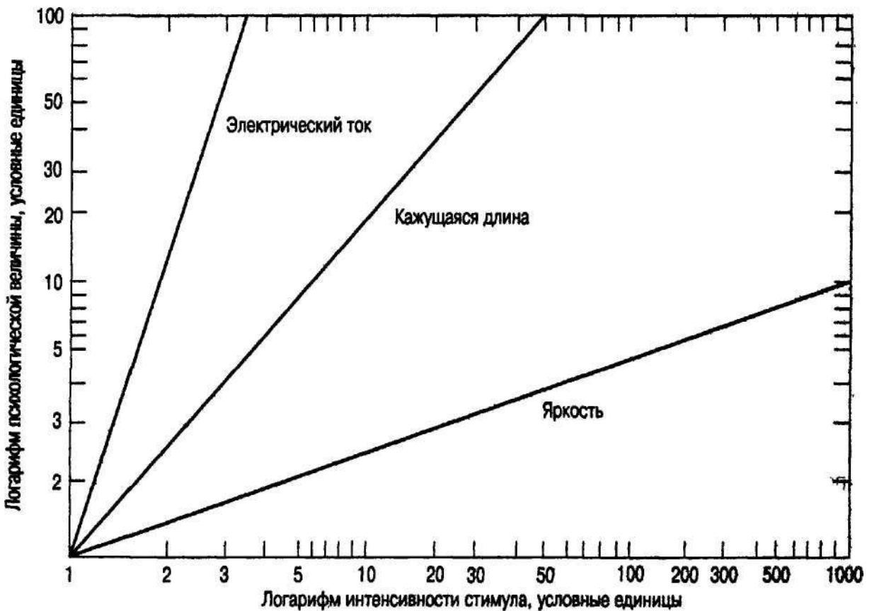
Рис. 2.11. Степенные функции, отложенные в логарифмических координатах
