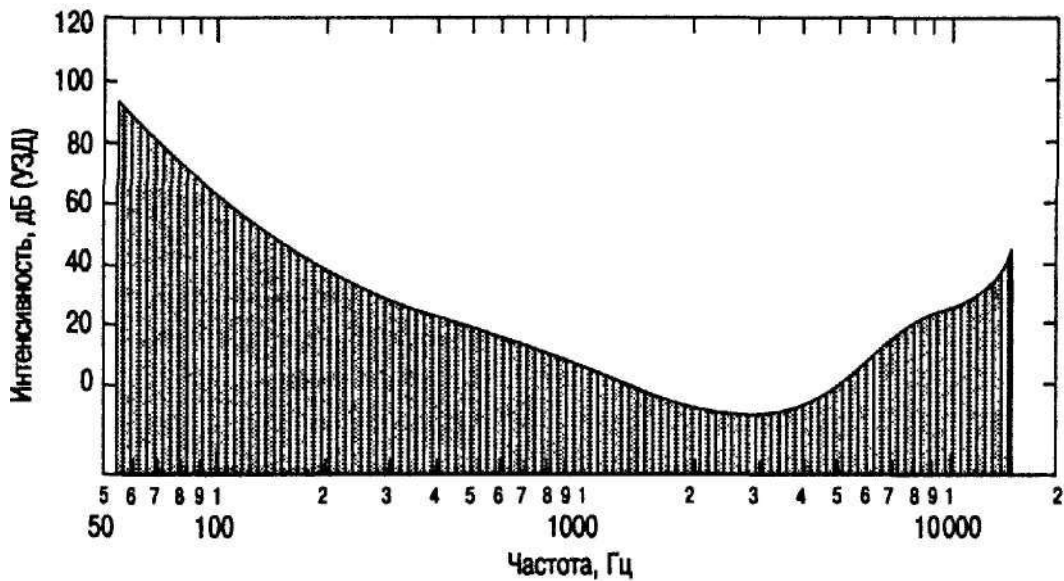
Рис. 13.1. Слуховой порог как функция частоты
