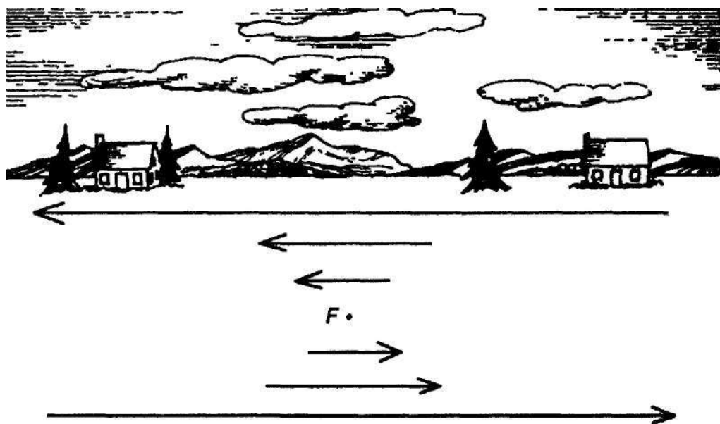
Рис. 9.16. Схема параллакса движения
