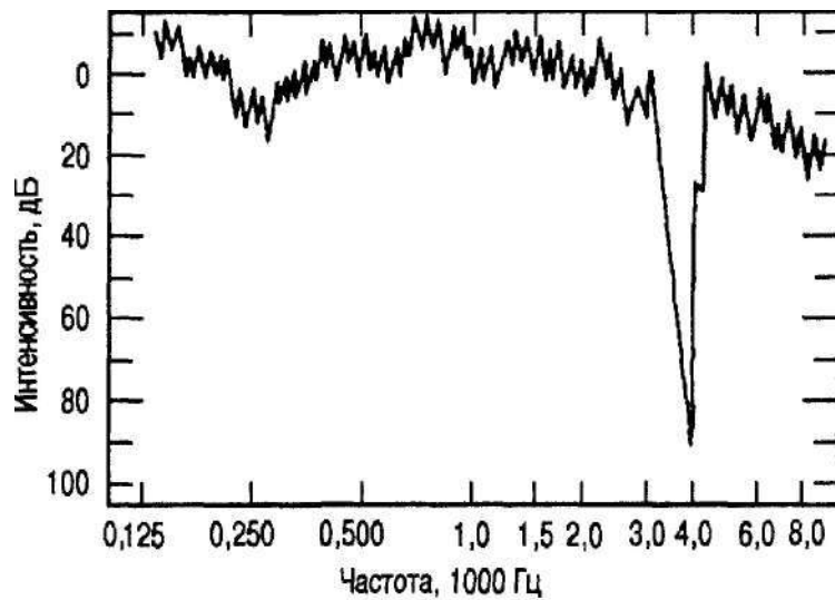
Рис. 12.23. Аудиометрическая функция, полученная по методу Бекеша, или методу слежения Кривая отражает зависимость порога интенсивности от частоты. Тональный пробел - свидетельство того, что испытуемый не слышит звуки, частота которых равна приблизительно 4000 Гц
